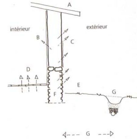
^ Tableau des principaux principes préventifs liés à l'eau Source: Terre Crue, B. PIGNAL p 44
