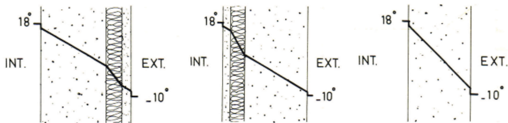
L'isolation par l'extérieur empêche les migrations de vapeur d'eau entre le milieu extérieur et le pisé.
