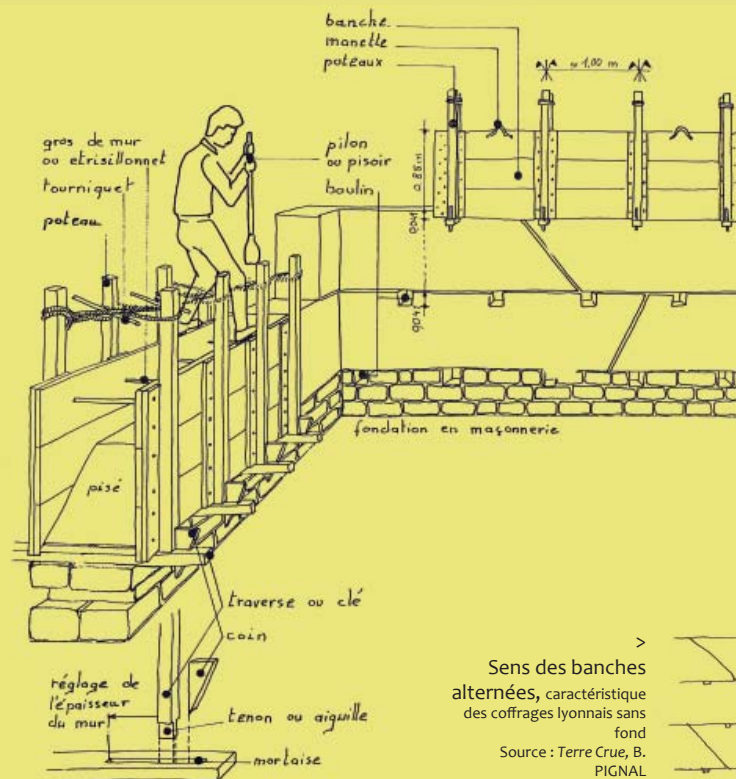
< Technique de mise en œuvre Source : Le Bâti ancien en lyonnais
