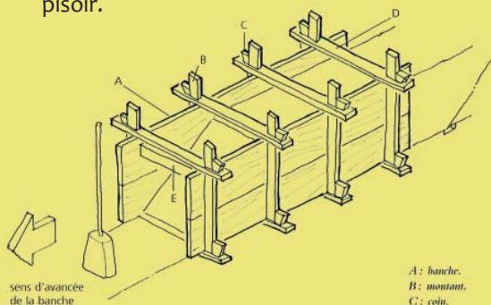
^ La banche lyonnaise Source : Terre Crue, B. PIGNAL
