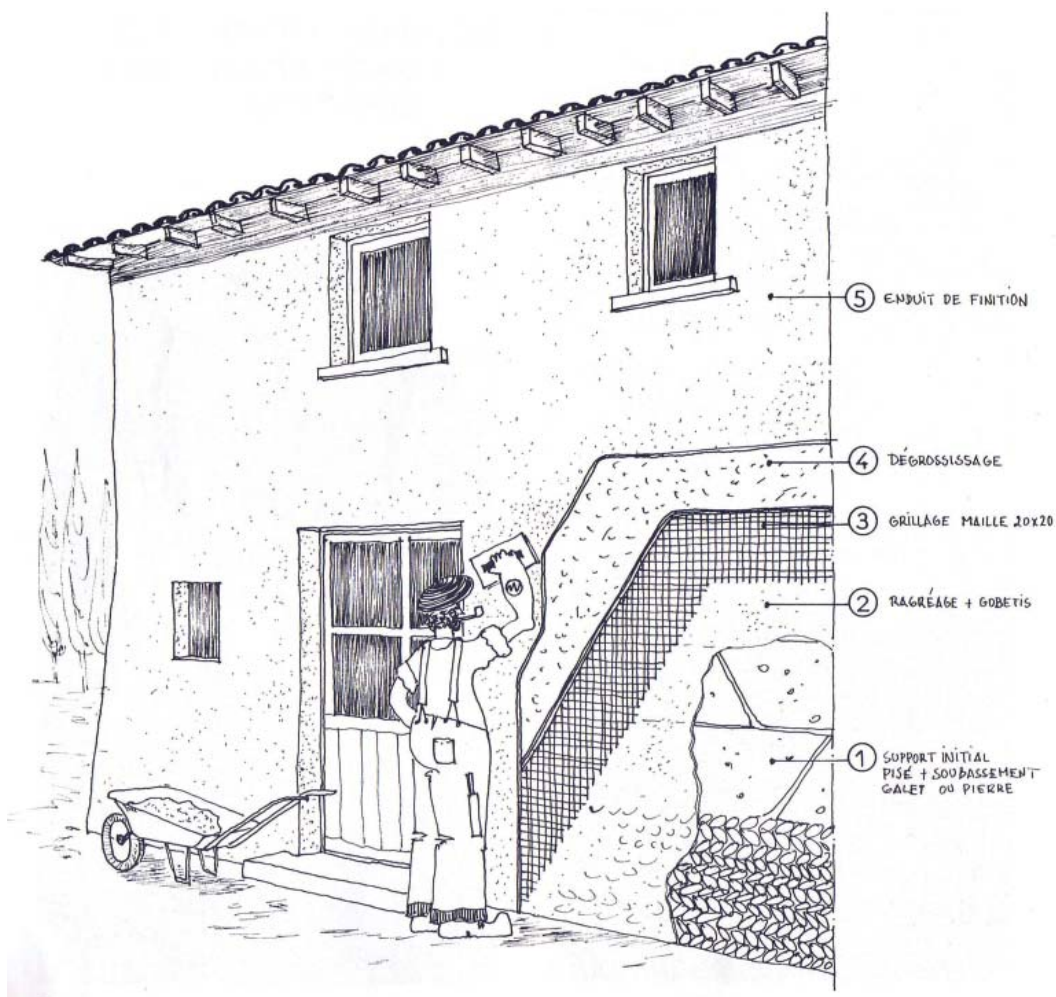
^ Dessin de réfection d'un enduit Source: Le Bâti ancien en lyonnais, p 86
