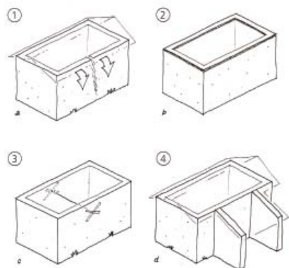
1 Comment stabiliser un mur en pisé Source: Terre Crue, B. PIGNAL p 47
